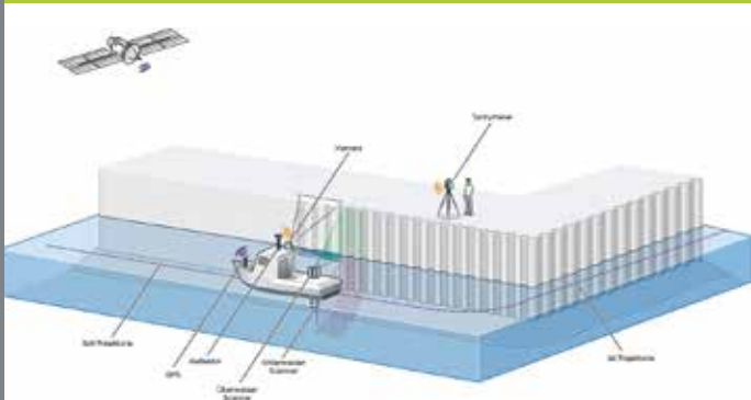
Multi-Sensor-Plattform zur Erfassung von Hafeninfrastrukturen
