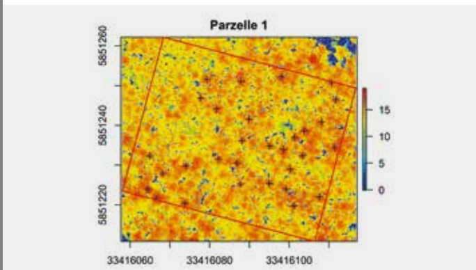
Baumhöhenermittlung aus Laserscandaten
